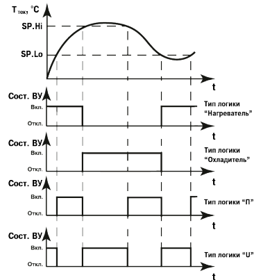
Рисунок 7.1 – Типы логики работы прибора
