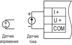
Рисунок 5.5 – Схемы подключения входных сигналов
