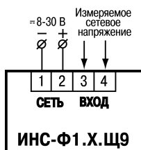
Рисунок 7 – Назначение клеммника прибора модификации Ш9
