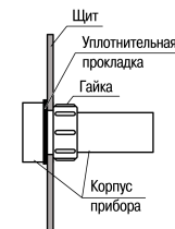
Рисунок 3 – Монтаж прибора щитового крепления
