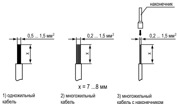
Рисунок 5 – Требования к сечениям жил кабелей
