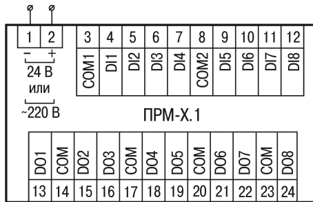
Рисунок 3 – Назначение контактов клемника
