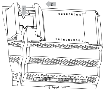
Рисунок 5 – Укладка шлейфа в углубление
