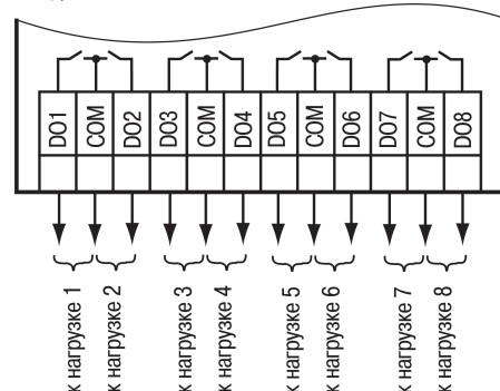
Рисунок 9 – Схема подключения нагрузки к ВЭ типа «Р»
