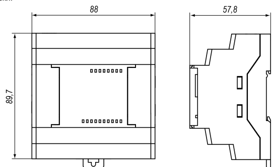
Рисунок 2 – Габаритные размеры
