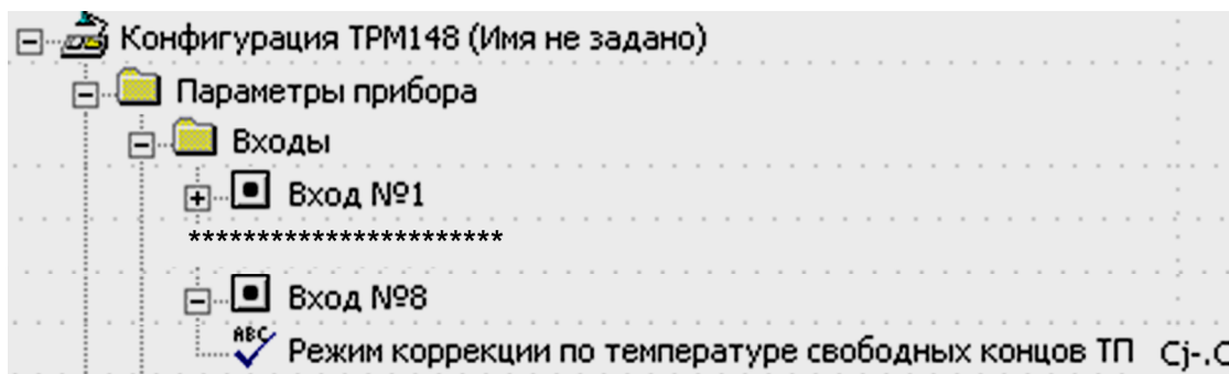
Рисунок 10.8 – Конфигуратор. КХС
