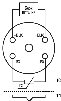
Рисунок 6.2 – Подключение прибора
