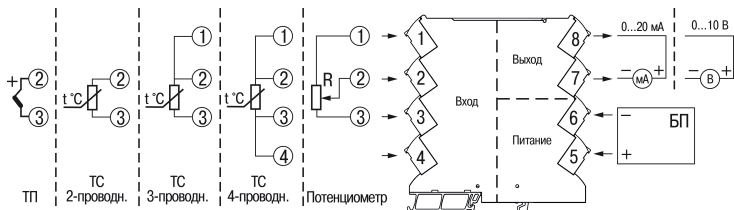
Рисунок 6.3 – Подключение прибора
