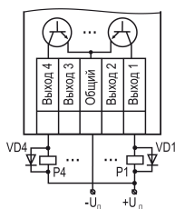
Рисунок 9 – Подключение нагрузки к ВЭ типа «К»
