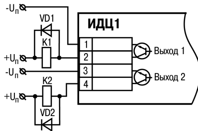
Рисунок 5.4 – Схема подключения реле к прибору
