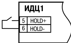
Рисунок 5.5 – Схема подключения коммутирующего устройства к прибору
