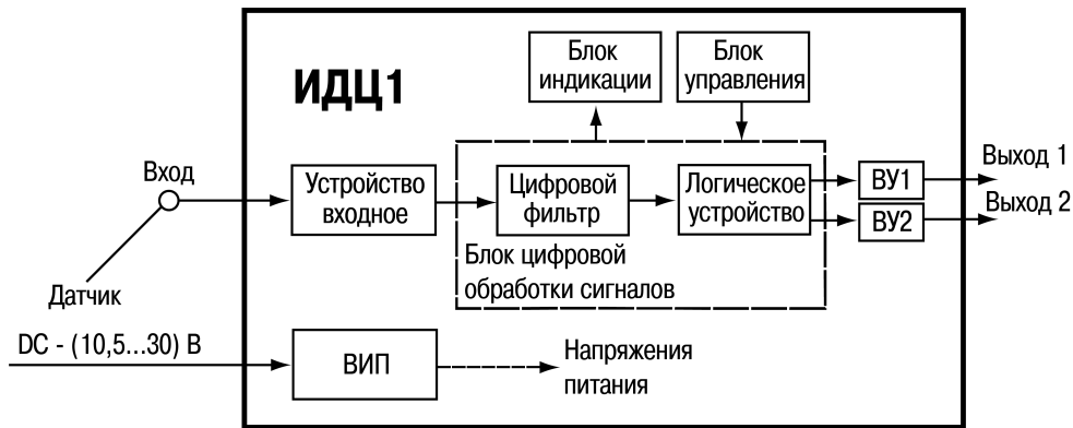
Рисунок 6.1 – Функциональная схема прибора
