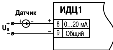
Рисунок 5.2 – Схема подключения к прибору датчика с сигналами постоянного тока от 0 до 5 мА, от 0 до 20 мА, от 4 до 20 мА
