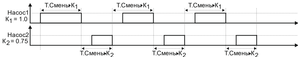
Рисунок 3.6 - Работа насосов при различных коэффициентах хода
