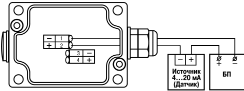
Рисунок 4 – Подключение справа
