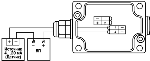
Рисунок 5 – Подключение слева
