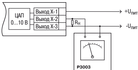
Рисунок 8.8 – Подключение ВУ1 типа И ( R_n = 500 \text{ Ом} )
