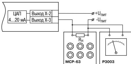
Рисунок 8.9 – Подключение ВУ1 типа У
