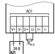
Рисунок 11 – Схема подключения к АО ПРМ-х.3 нагрузки типа У
