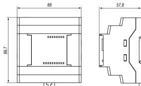
Рисунок 2 – Габаритные размеры
