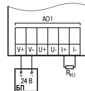
Рисунок 10 – Схема подключения к АО ПРМ-х.3 нагрузки типа И
