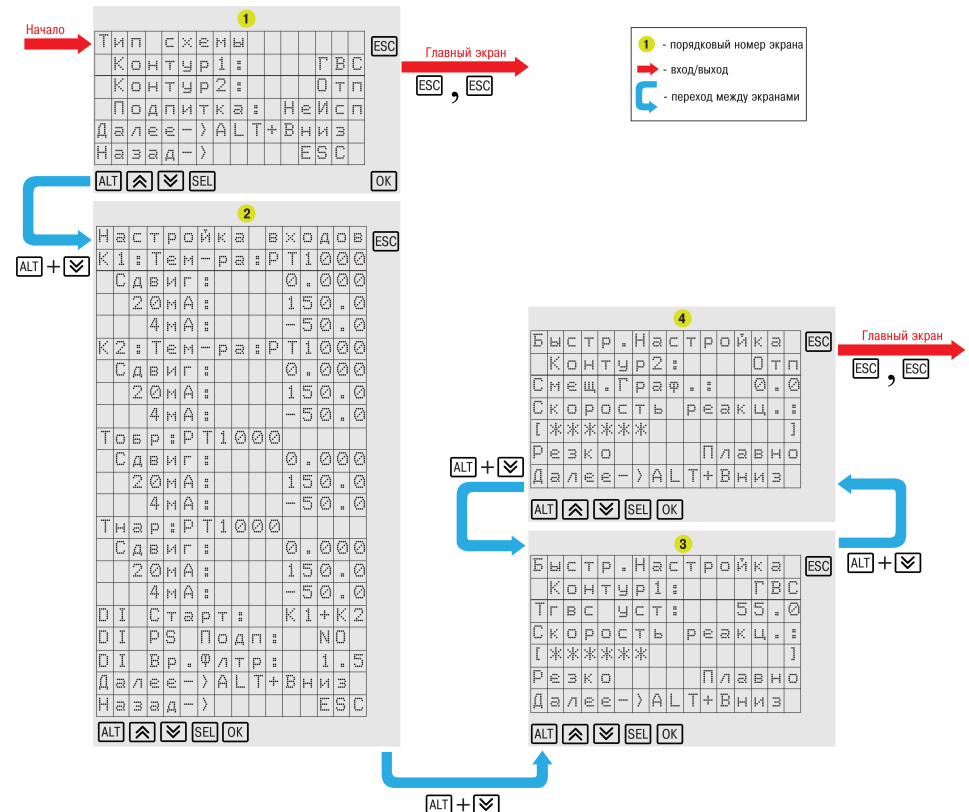
Рисунок 10.2 – Схема первичной настройки
