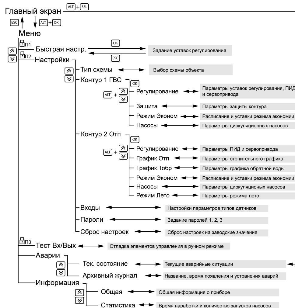
Рисунок 9.4 – Схема переходов по меню
