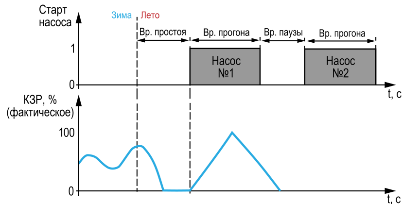
Рисунок 12.11 – Прогон при сезоне «Лето»
