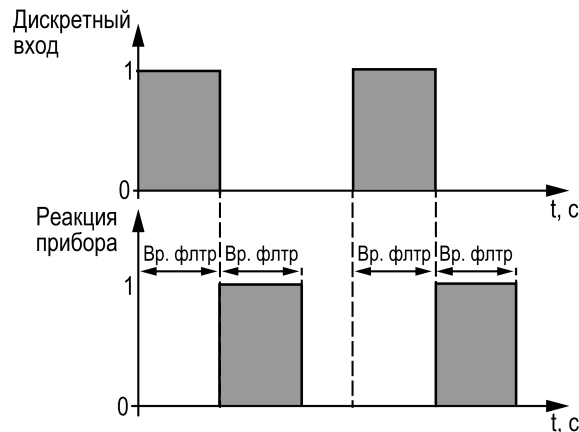
Рисунок 10.5 – Принцип работы времени фильтрации
