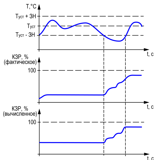
Рисунок 13.1 – Принцип работы КЗР
