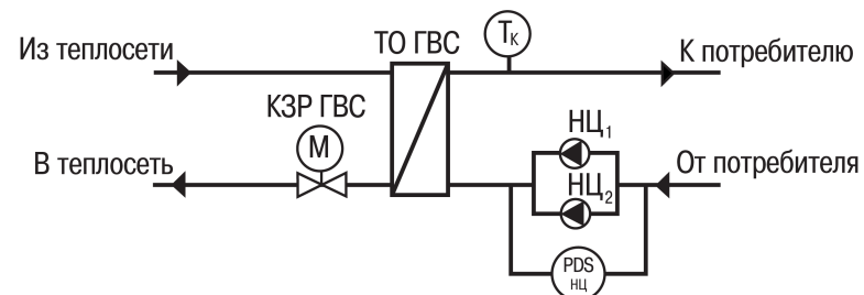
Рисунок 2.2 – Схема контура «ГВС»
