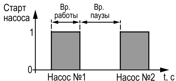
Рисунок 12.8 – Чередование насосов
