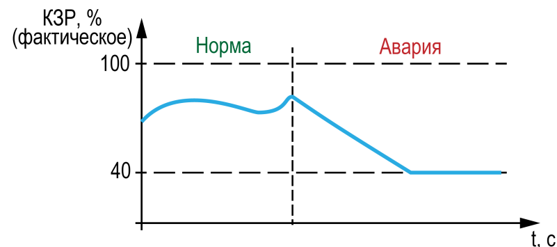
Рисунок 13.3 – Работа КЗР – норма/авария
