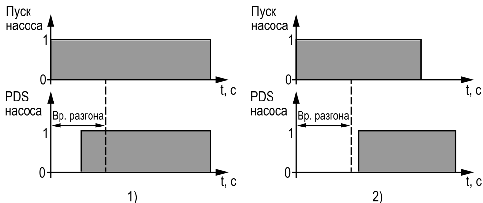
Рисунок 12.7 – Время разгона насоса: 1) нормальная работа, 2) во время аварии
