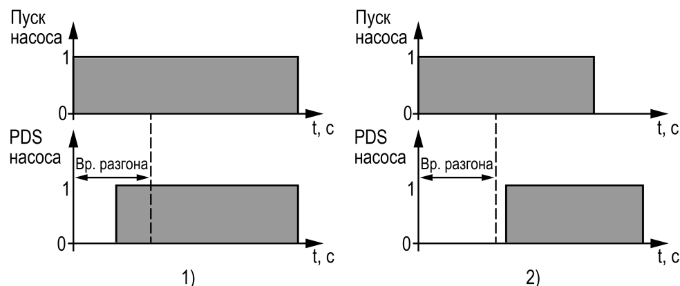
Рисунок 13.6 – Время разгона насоса: 1) нормальная работа, 2) во время аварии
