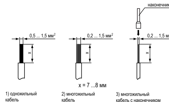
Рисунок 8.1 – Требования к сечениям жил кабелей
