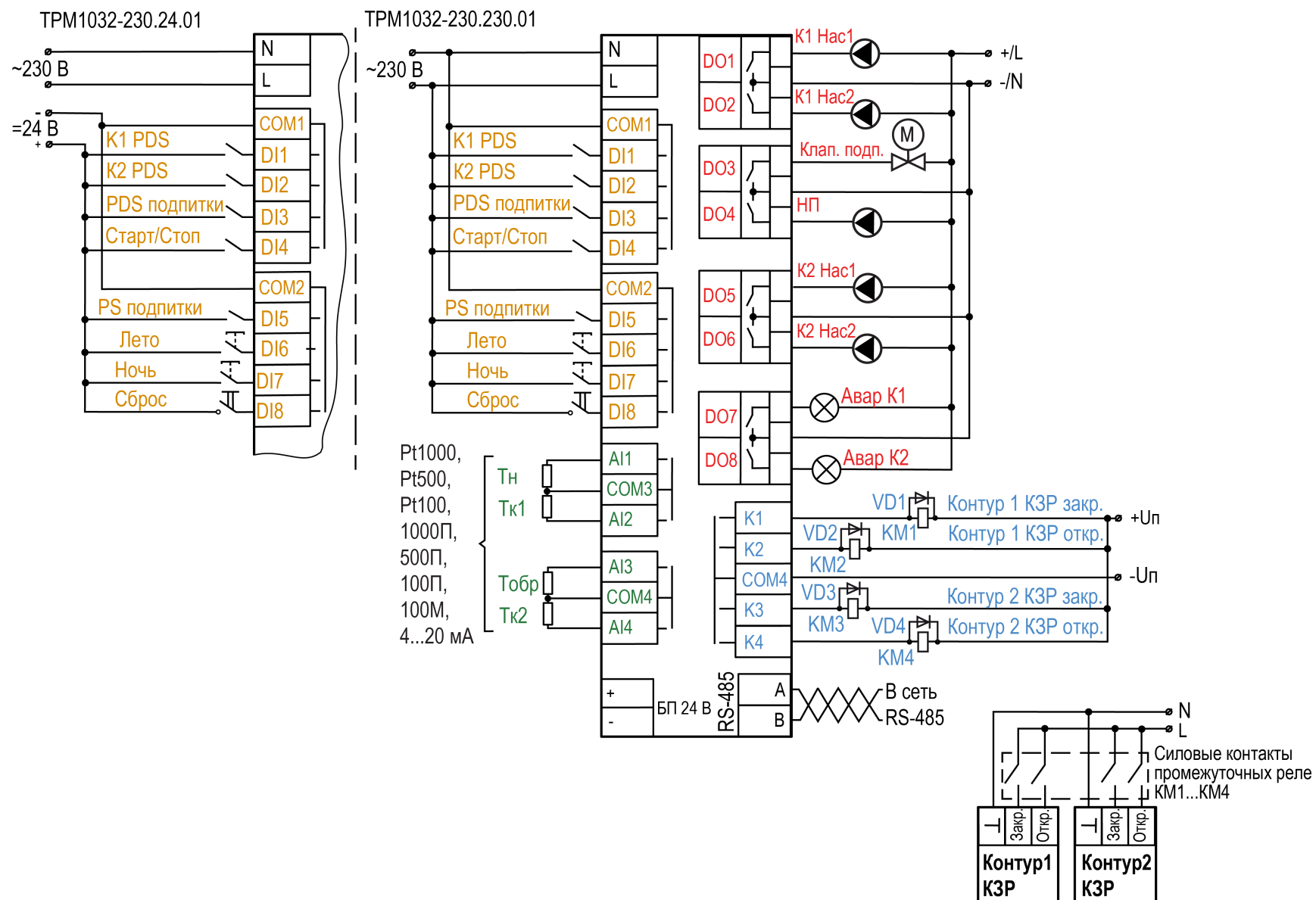
Рисунок 8.3 – Схема подключения
