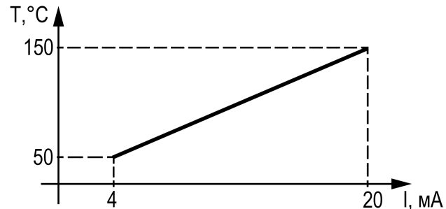
Рисунок 10.4 – Границы измерений датчика 4...20 мА
