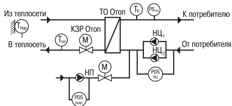
Рисунок 2.1 – Схема контура «Отопление»
