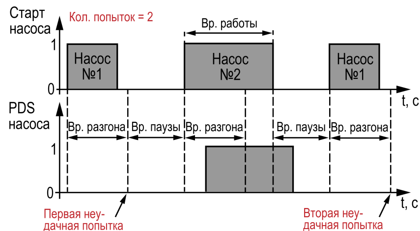
Рисунок 12.9 – Перезапуск насоса
