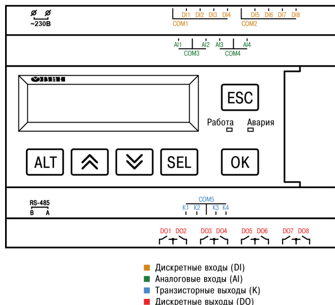
Рисунок 8.2 – Расположение и цветовая маркировка клемм
