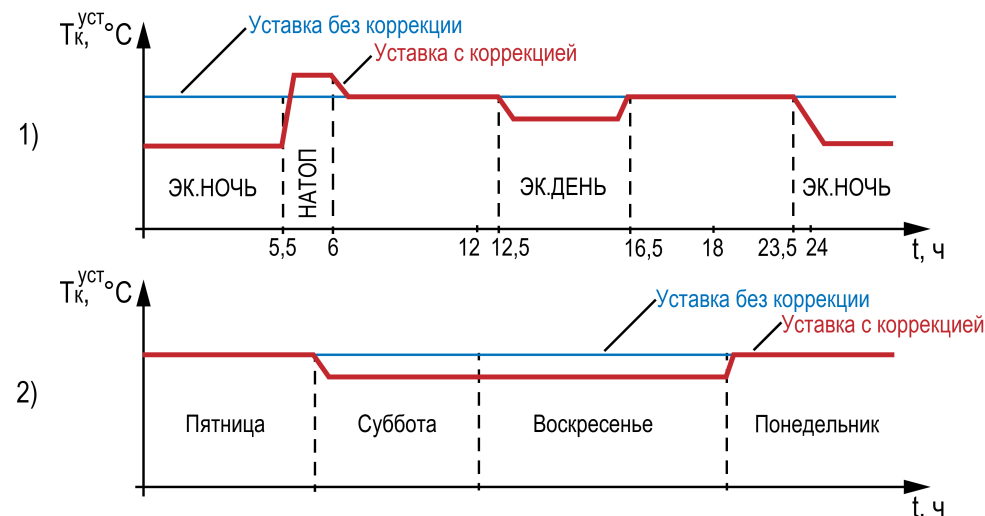
Рисунок 12.6 – Режим экономии: 1) в дневное время, 2) по выходным дням
