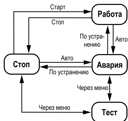
Рисунок 9.1 – Основные режимы работы
