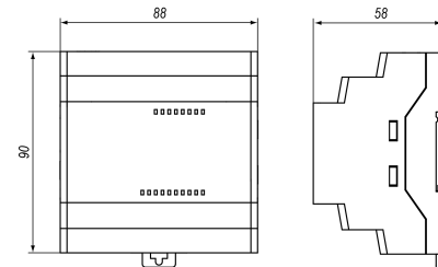
Рисунок 2 – Габаритные размеры
