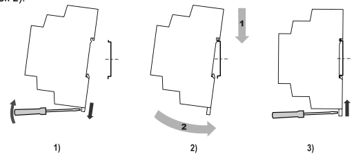
Рисунок 1 – Установка прибора
