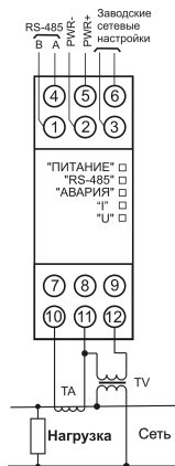
Рисунок 4 – Подключение прибора к однофазной сети через согласующие трансформаторы тока и напряжения
