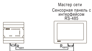
Рисунок 6 – Типовая схема подключения для PR100 в режиме Slave
