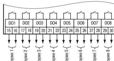
Рисунок 5 – Схема подключения нагрузки к ВЭ типа «Р»
