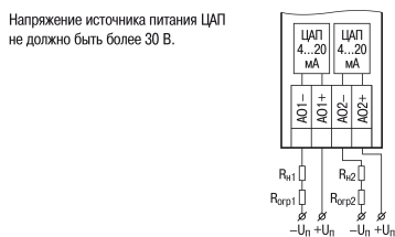
Рисунок 9 – Подключение нагрузки к ВЭ типа «I»
