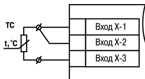
Рисунок 6.7 – Трехпроводная схема подключения ТС
