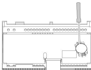
Рисунок 10.2 – Замена батареек
