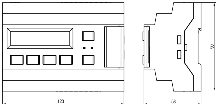
Рисунок 2 – Габаритный чертеж прибора
