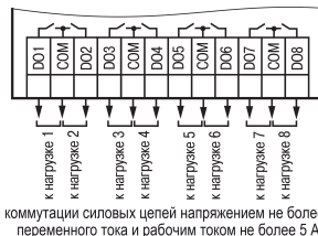
Рисунок 8 – Подключение нагрузки к ВЭ типа «Р»
