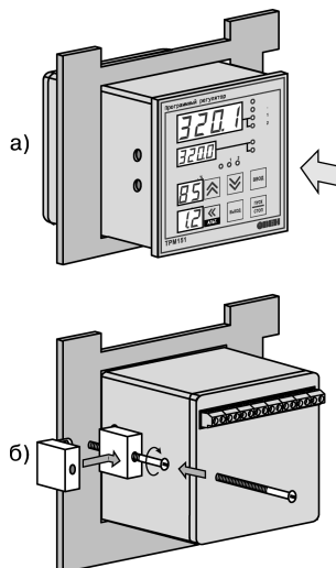
Рис. 7.2 – Установка прибора щитового крепления
