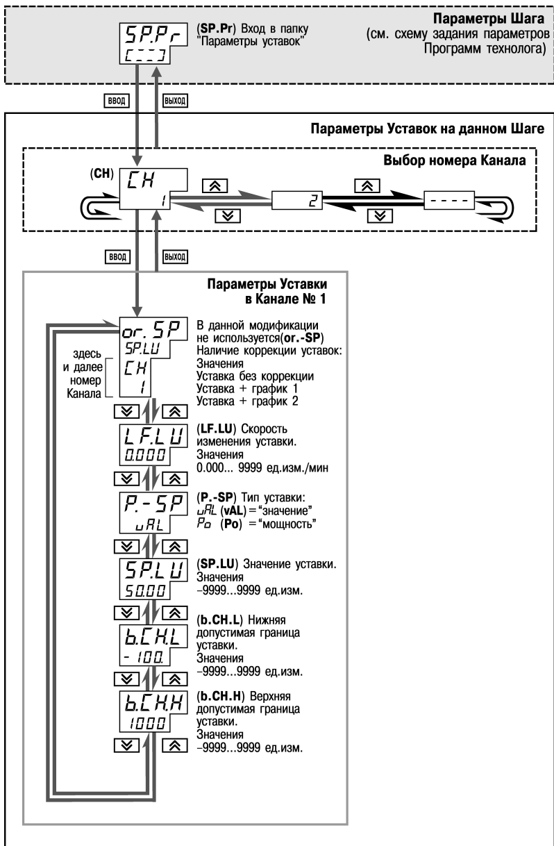
Рисунок 11.16 – Схема задания параметров Программ технолога и Устроек (продолжение). Задание параметров Устроек на данном Шаге Программы
