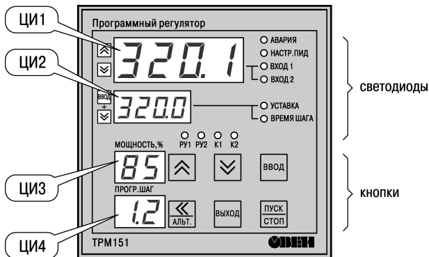
Рисунок 5.1 – Лицевая панель прибора
