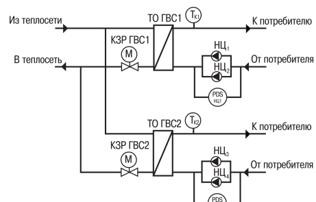
Рисунок 6 – Схема контура «ГВС + ГВС»
