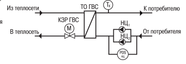
Рисунок 3 – Схема контура «ГВС»
