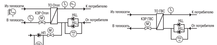
Рисунок 3 – Схема контура «ГВС»
