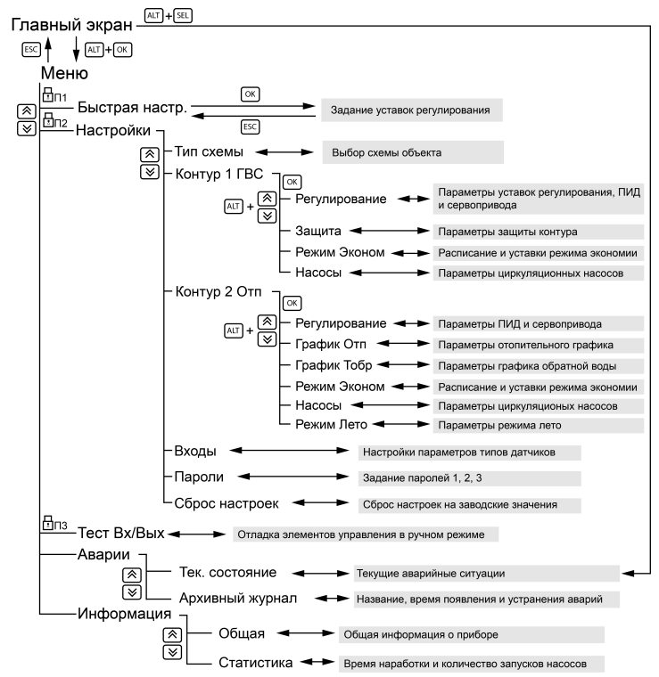
Рисунок 9 – Схема переходов по меню
