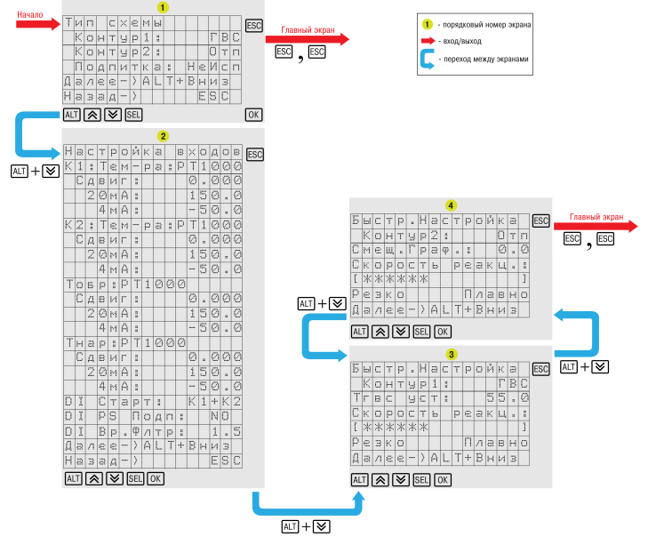
Рисунок 10 – Схема первичной настройки
