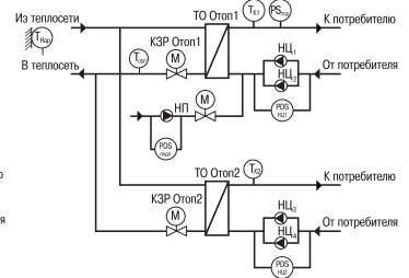
Рисунок 5 – Схема контура «Отопление + отопление»
