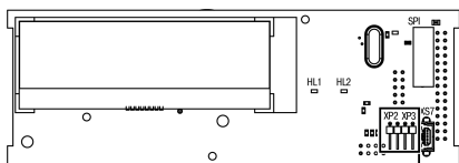
Рисунок 4 – Схема настройки AI1...AI4
