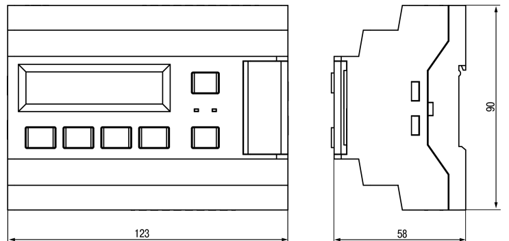
Рисунок 2 – Габаритный чертеж прибора
