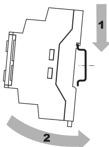
Рисунок 4.1 – Монтаж
