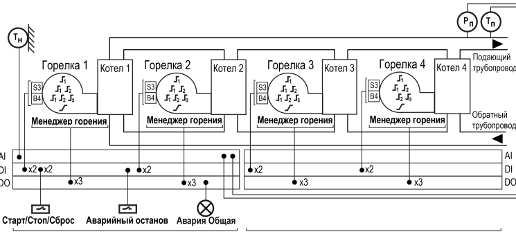
Рисунок 6.1 – Объект управления
