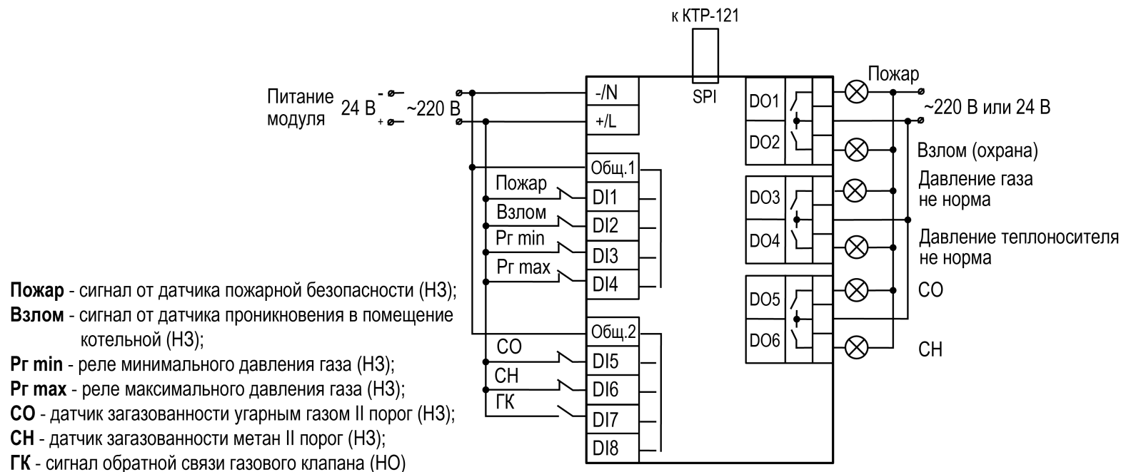
Рисунок 6.5 – Схема подключения к ПРМ-1 сигналов общекотельных аварий
