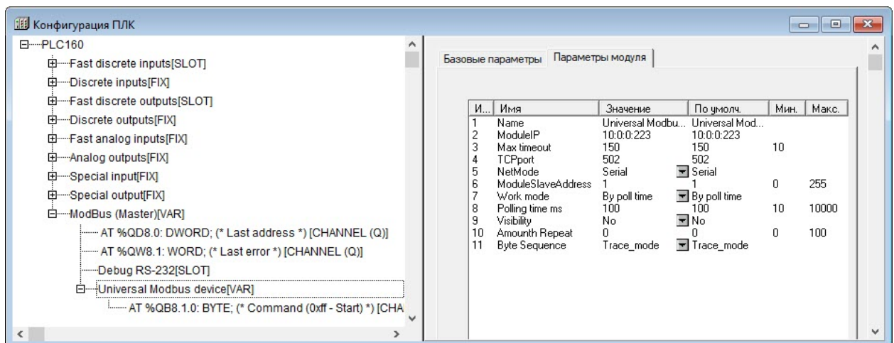
Рисунок 10.24 – Параметры подмодуля Universal ModBus device
