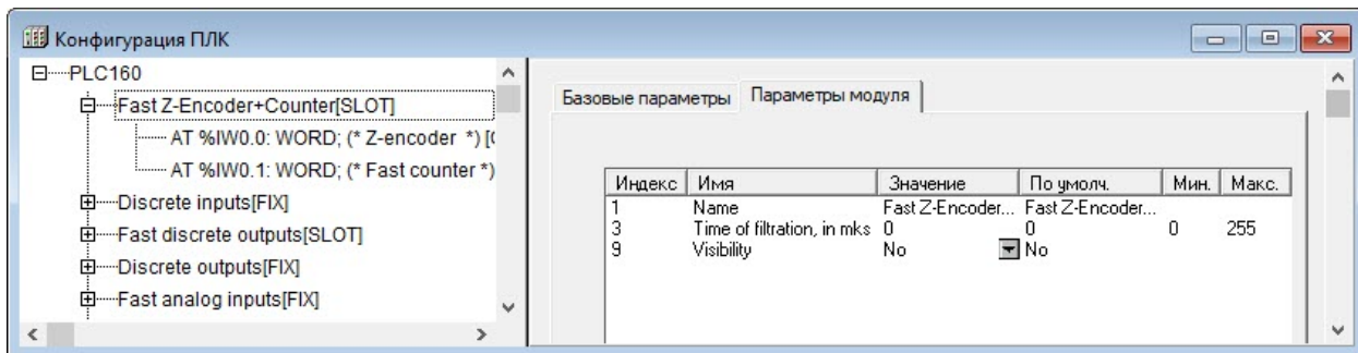
Рисунок 10.15 – Параметры модуля «Высокочастотный Z-энкодер + счетчик»
