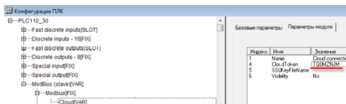
Рисунок 13.9 – Ввод токена OwenCloud в конфигурацию ПЛК
