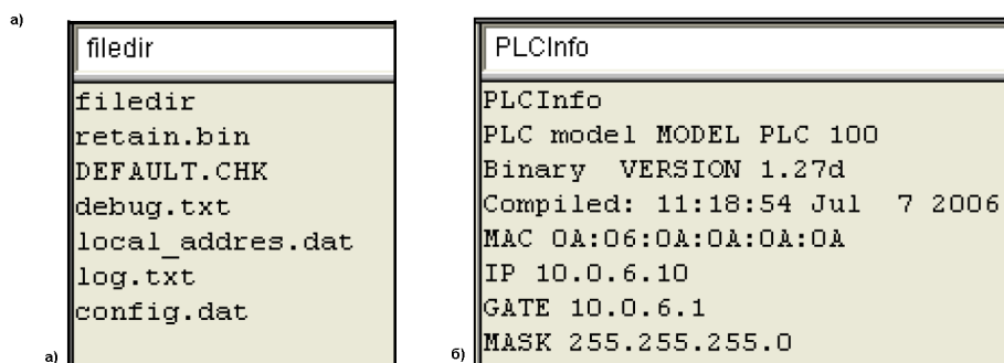
Рисунок 12.2 – Ввод команд (а) и реакция контроллера (б)
