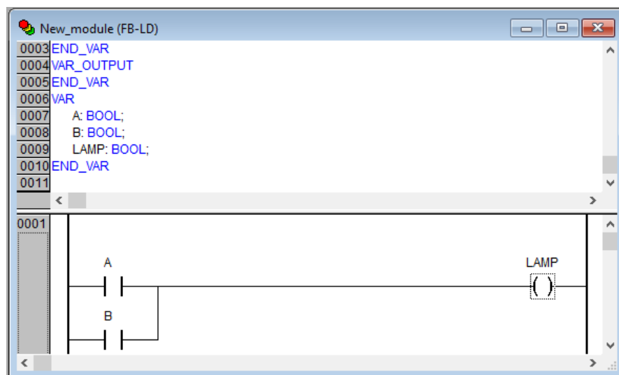
Рисунок 7.20 – Пример кода нового программного компонента
