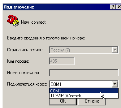
Рисунок 15.2 – Окно «Подключение»
