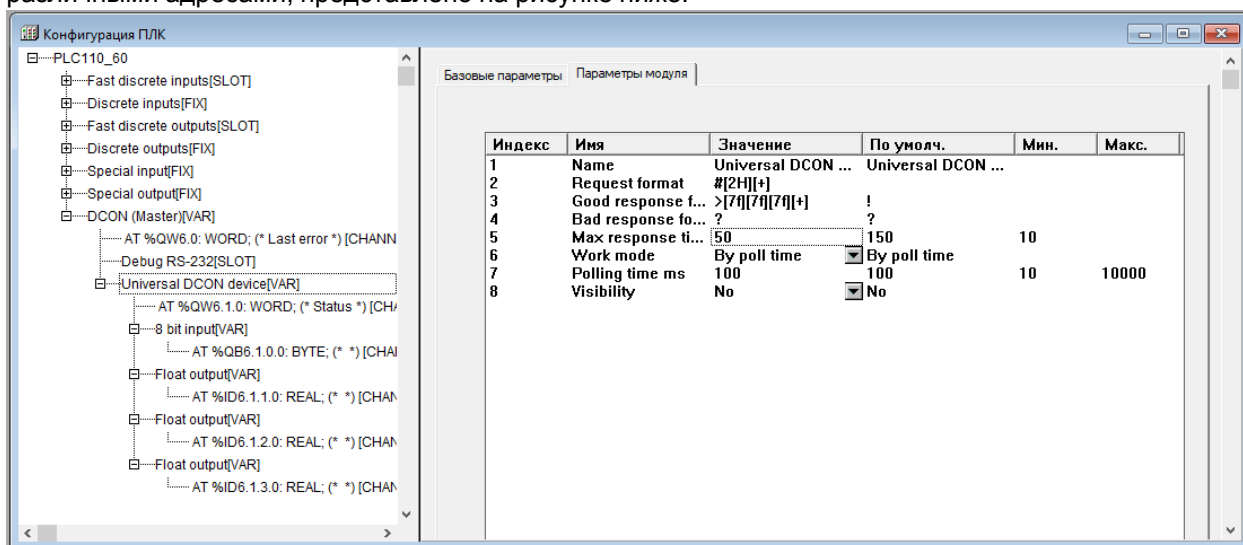
Рисунок Б.1 – Параметры подмодуля «Universal DCON device» модуля «DCON (Master)» для опроса входов модулей IPC-7033
