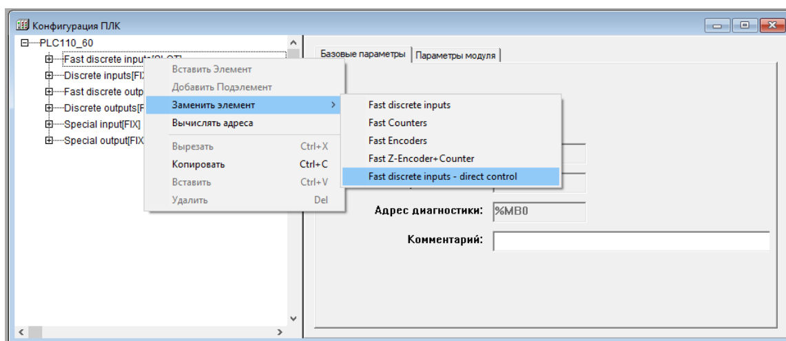
Рисунок 14.3 – Замена модуля
