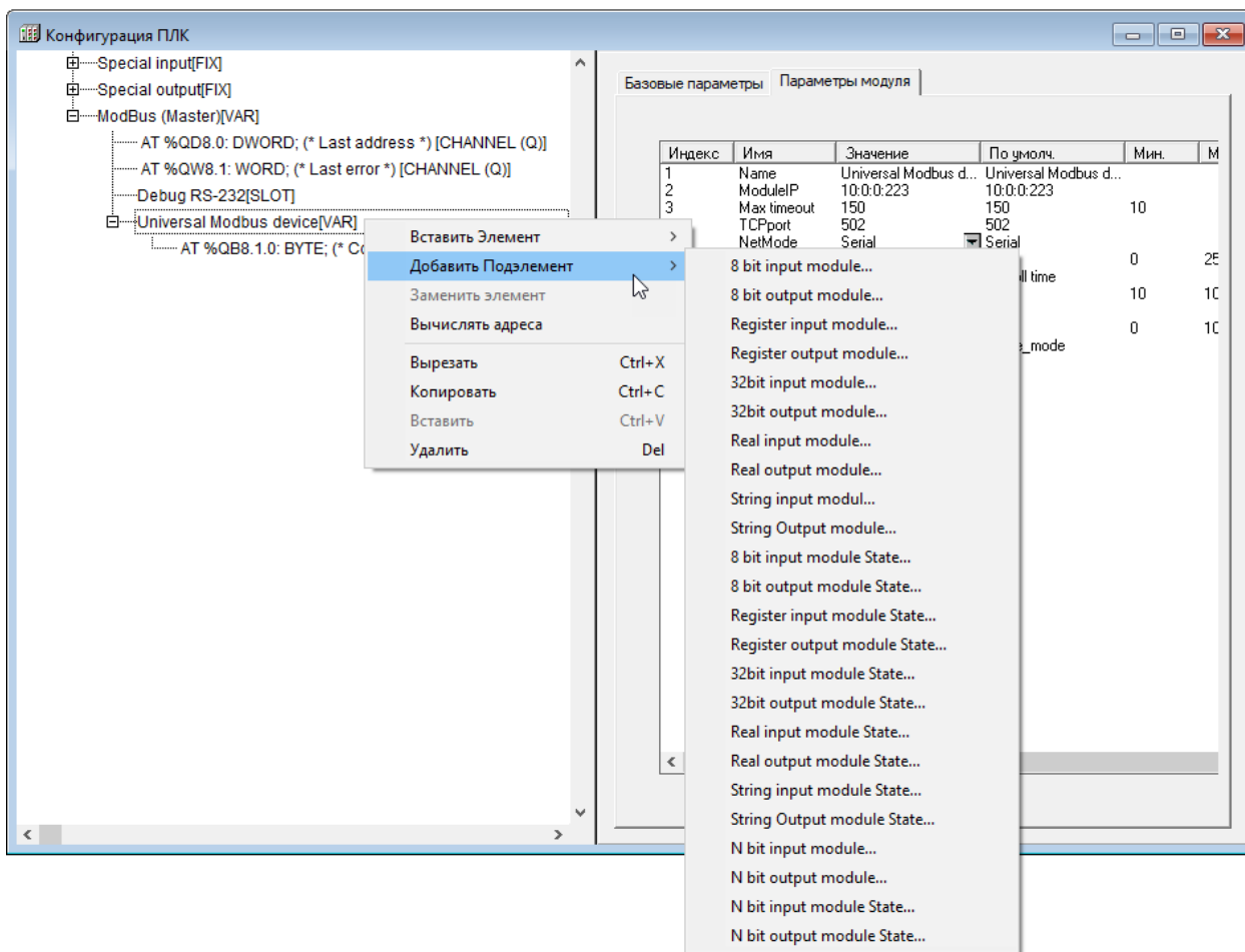
Рисунок 10.25 – Добавление каналов ввода-вывода подмодуля Universal Modbus device
