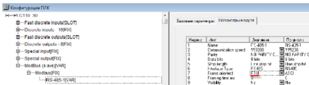
Рисунок 13.14 – Настройки интерфейса RS-485
