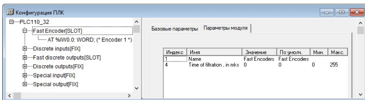
Рисунок 10.13 – Параметры модуля Высокочастотный энкодер (FastEncoder) для ПЛК110-32
