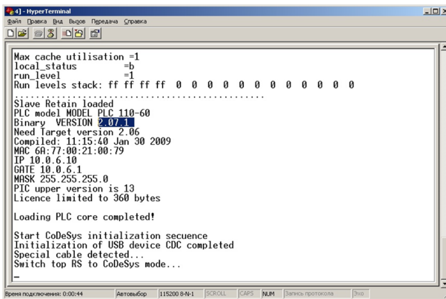
Рисунок 15.4 – Окно «HyperTerminal»
