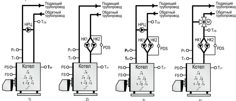
Рисунок 6.1 – Объект управления
