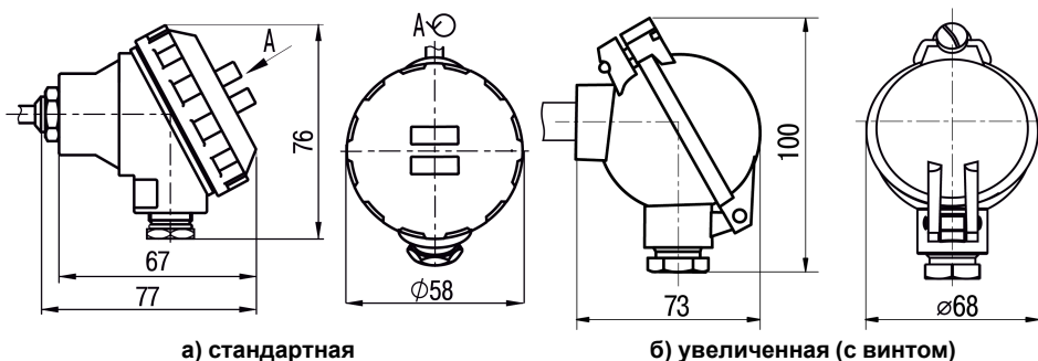
Рисунок Г.2 – Габаритные размеры металлической коммутационной головки
