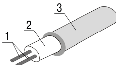
Рисунок 4.3 – Конструкция ЧЭ на основе КТМС
