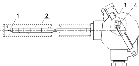
Рисунок 4.1 – Конструкция датчика с коммутационной головкой
