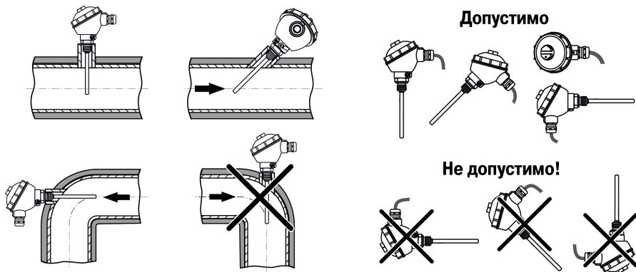
Рисунок 6.3 – Монтаж датчика с коммутационной головкой
