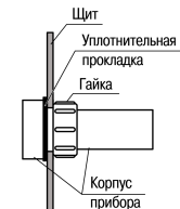
Рисунок 1 – Монтаж прибора щитового крепления
