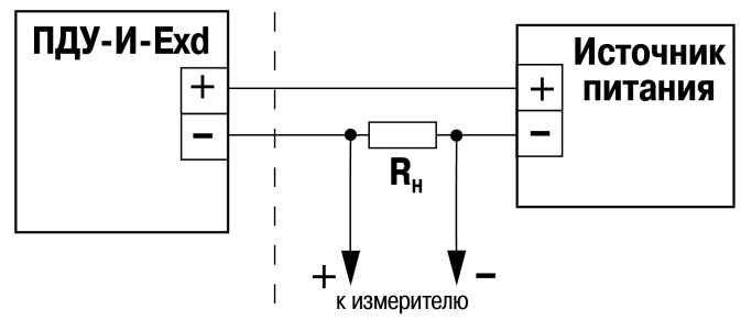
Рисунок 6.4 – Схема подключения
