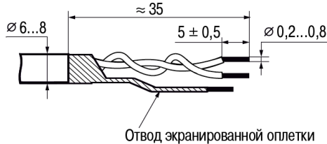
Рисунок 6.1 – Подготовка кабеля
