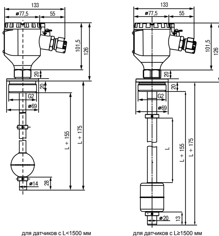
Рисунок 5.1 – Габаритные и присоединительные размеры
