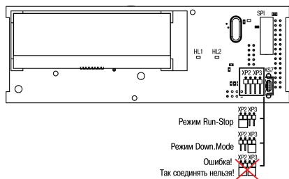
Рисунок 4 – Вид на верхнюю плату со снятой крышкой
