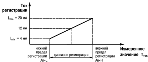
Рисунок 7.6 – Настройка диапазона в случае A_{п.L} < A_{п.H}
