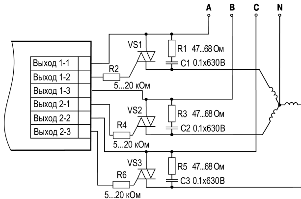
Рисунок 5.16 – Схема подключения силового симистора к ВУ типа СЗ
