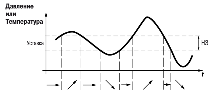
Рисунок 8.3 – Регулирование холодопроизводительности
