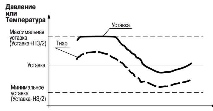
Рисунок 8.6 – График регулирования
